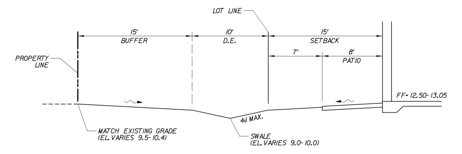
SECTION "B" N.T.S.
